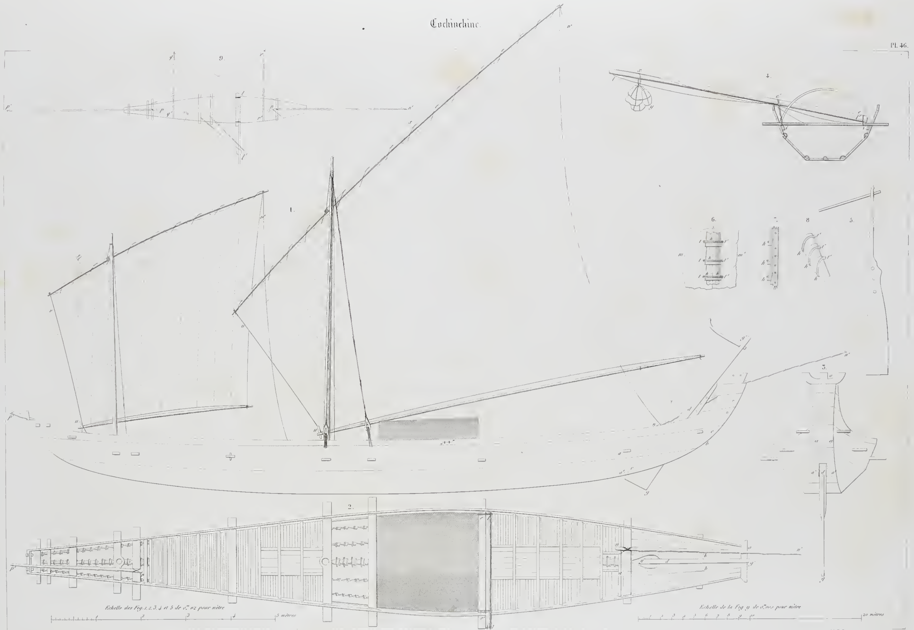
1. Gay-you, bateau de pêche de la baie de Tourane 2. Plan. 3. Elevation de l'arrière 4. Section par le mât principal 5. Gouvernail. 6 et 8. Détails de la couture des bordages 9. Disposition des arcs-boutants pour tenir les piquets
