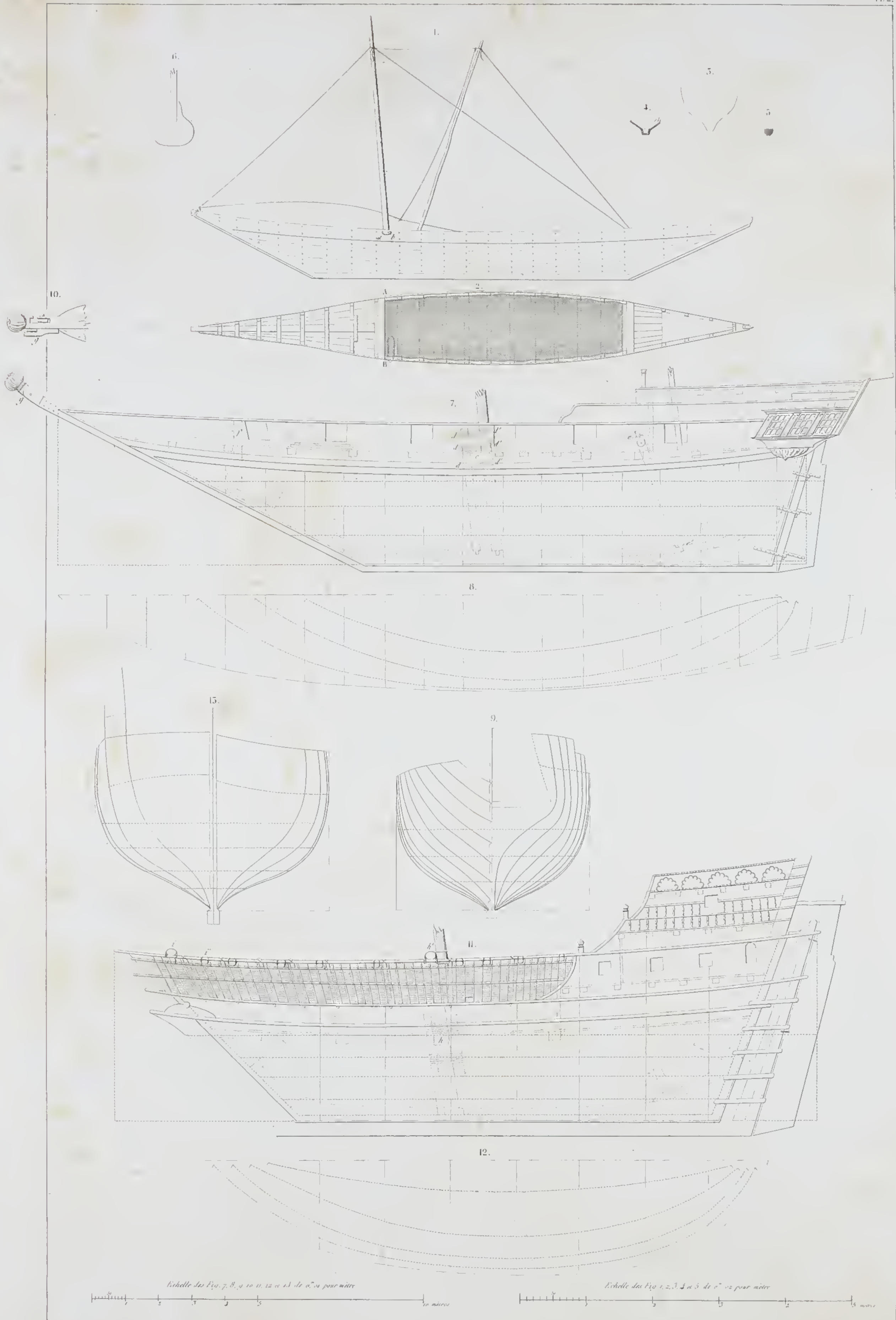
1. Bateau de Pêche de Hérak. 2. Plan. 3. Section verticale en AB. 4. Section de la Quille. 5. Section de l'Étrave et de l'Émbarcadere. 6. Ruyau (Hérak). 7. Daggali. 8. Plan. 9. Section. 10. Plan du haut de l'Étrave. 11. Daggali du Golfe de Calcutta. 12. Plan. 13. Section.
