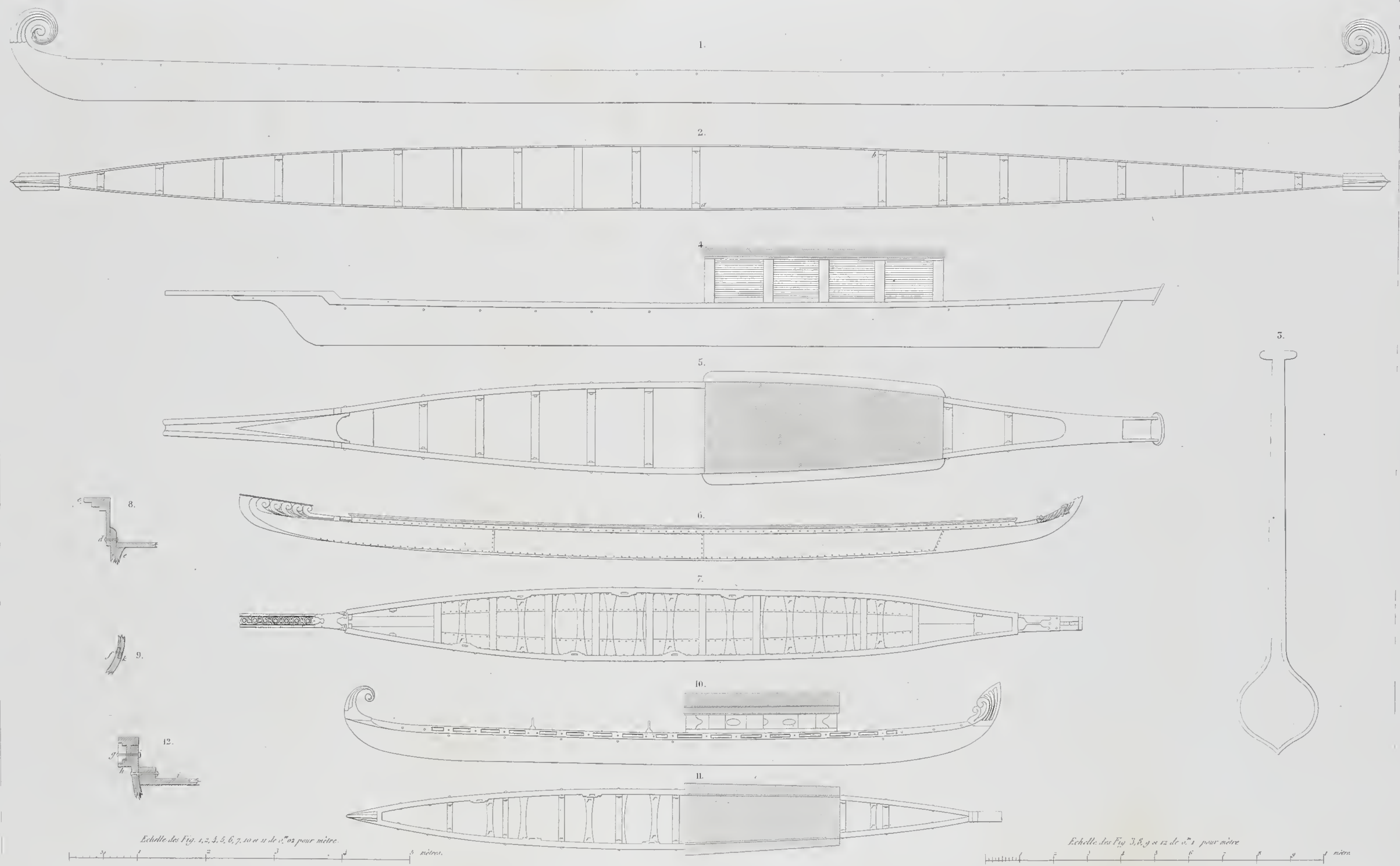
1. Pamban manchi ou bateau serpent du Sultan de Travancore. 2. Plan. 3. Dugais. 4. Woodie manchi de voyage. 5. Plan. 6. Woodie manchi de voyage. 7. Plan. 8. Section du plat bord. 9. Section des bords. 10. Pamban manchi. 11. Plan. 12. Section du plat bord.
