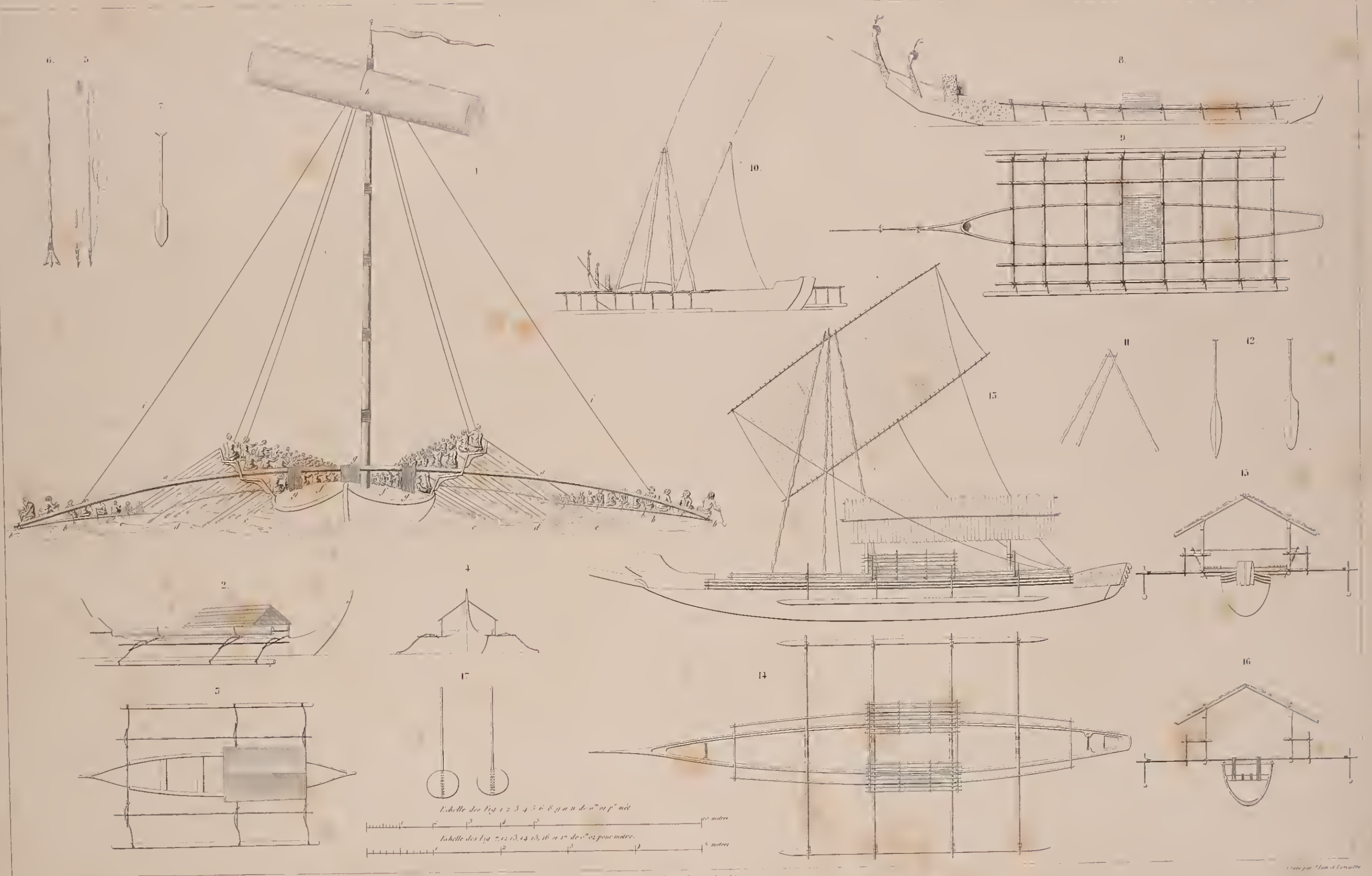
1. Vue de l'avant du navire à trois rangs de mâts nommé Pomanga 2. Pirogue de l'île Waigien 3. Plan 4. Élévation de l'avant 5. Mast pour les pirogues 6. Plan 7. Pirogue 8. Plan de pirogue du port Cerey 9. Plan 10. Vue perspective 11. Appareil des mâts 12. Pirogues 13. Pirogue du port Cerey 14. Plan 15. Élévation de l'arrière 16. Section par le milieu 17. Pirogue
