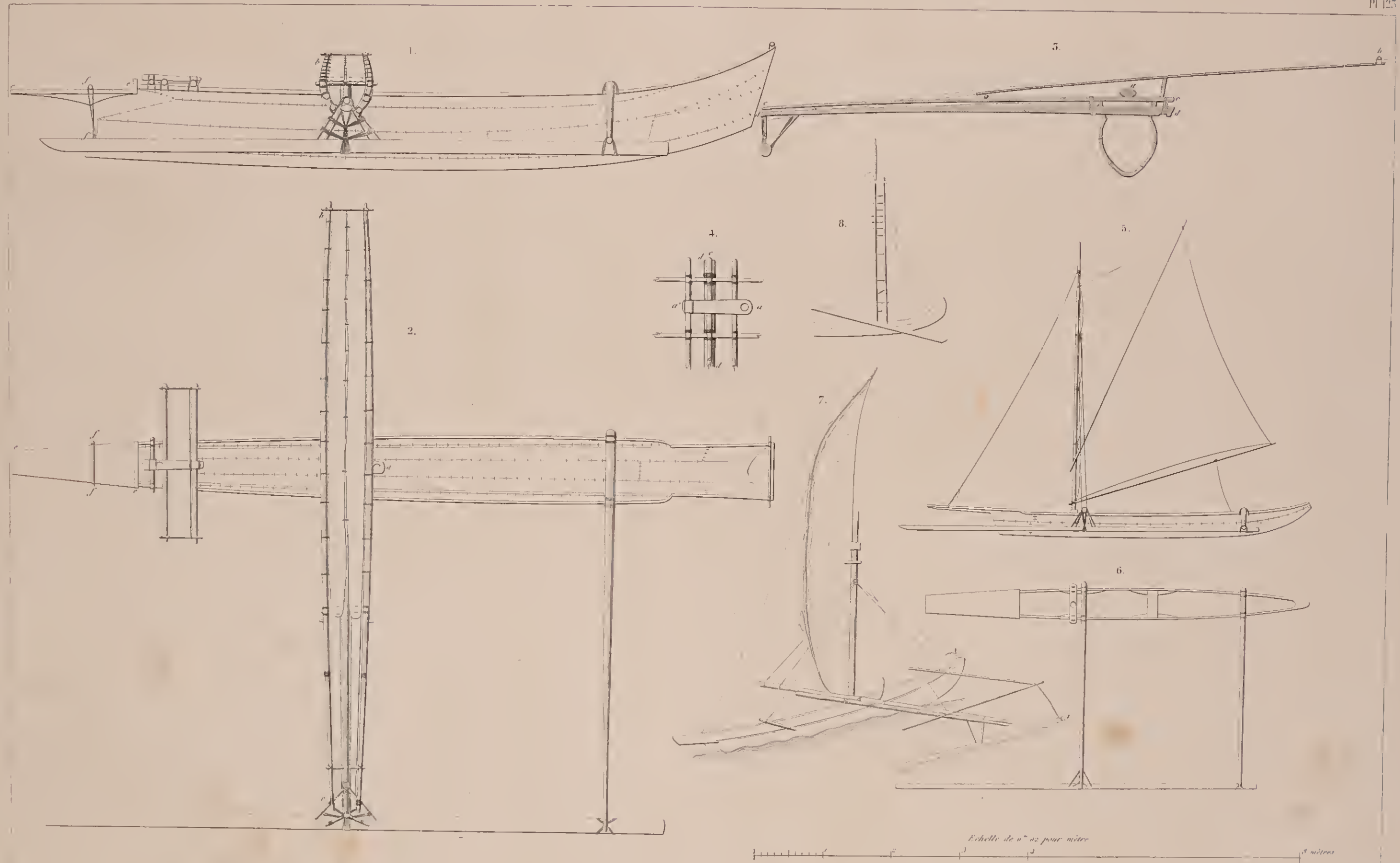
1. Grande Pirogue de Taïti 2. Plan 3. Section 4. Châssis qui réunit les deux côtés. 5. Petite Pirogue 6. Plan 7. Ancienne voile de Taïti 8. Ancien mât
