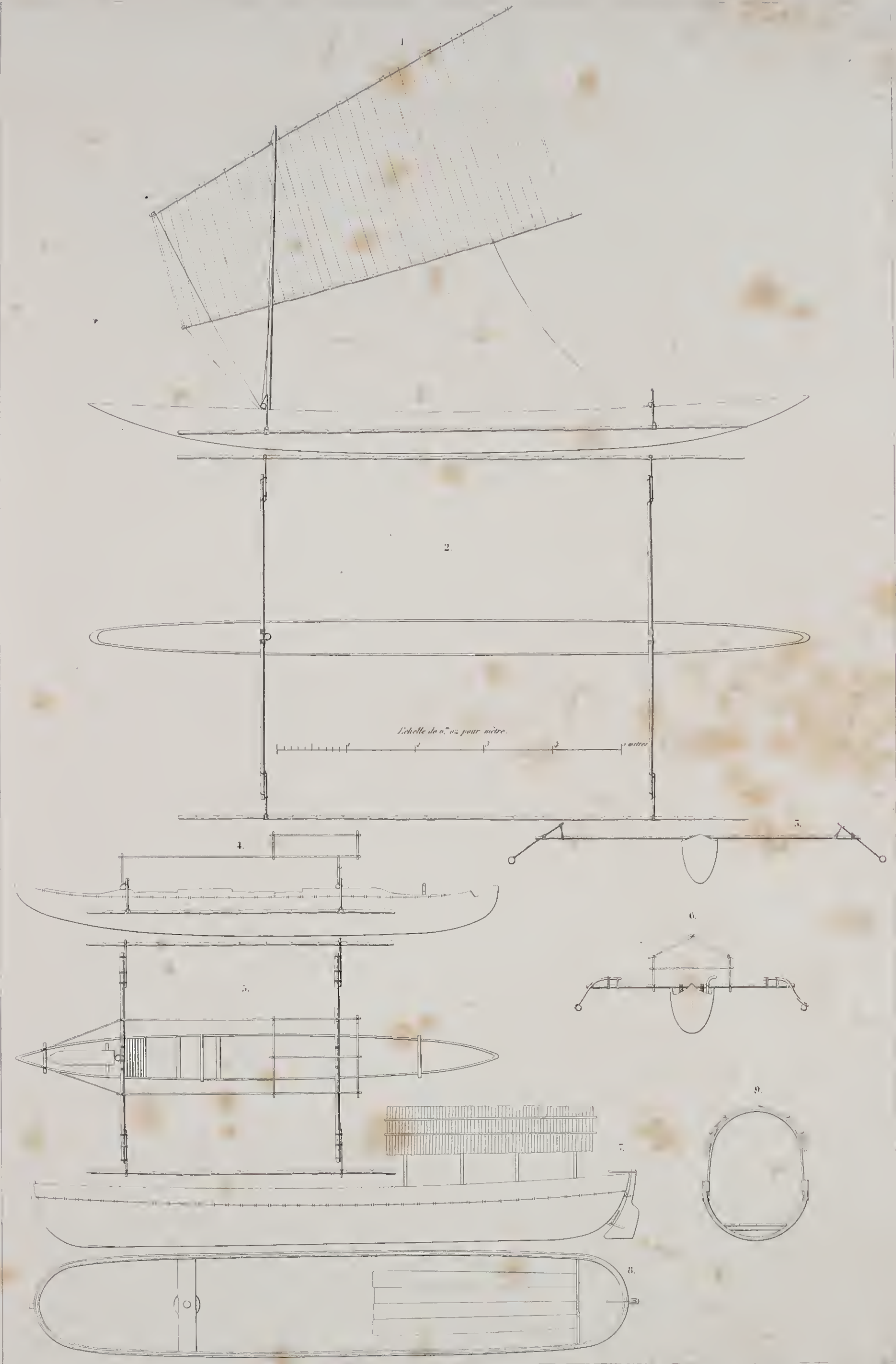
1. Vue de côté de la coque. 2. Plan. 3. Elevation de l'arrière. 4. Vue de côté de la coque. 5. Plan. 6. Elevation de l'arrière. 7. Vue de côté de la coque. 8. Plan. 9. Elevation de l'arrière.
