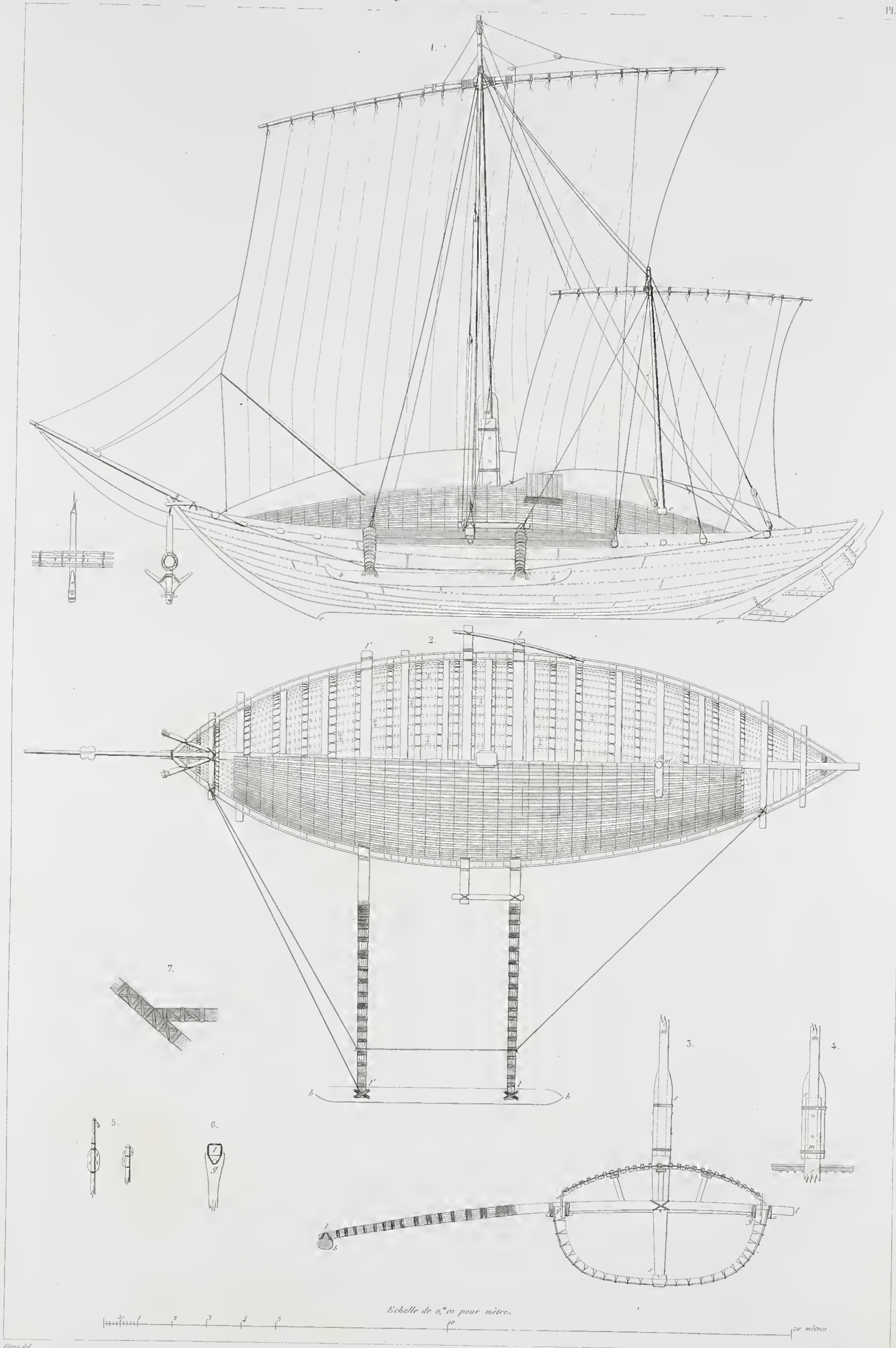
1. Demi à balancier 2. Plan 3. Section par le maître bau. 4. Profil du grand mât. 5. Tête des mâts 6. Grand levier et couple qui le soutient. 7. Ventouse
