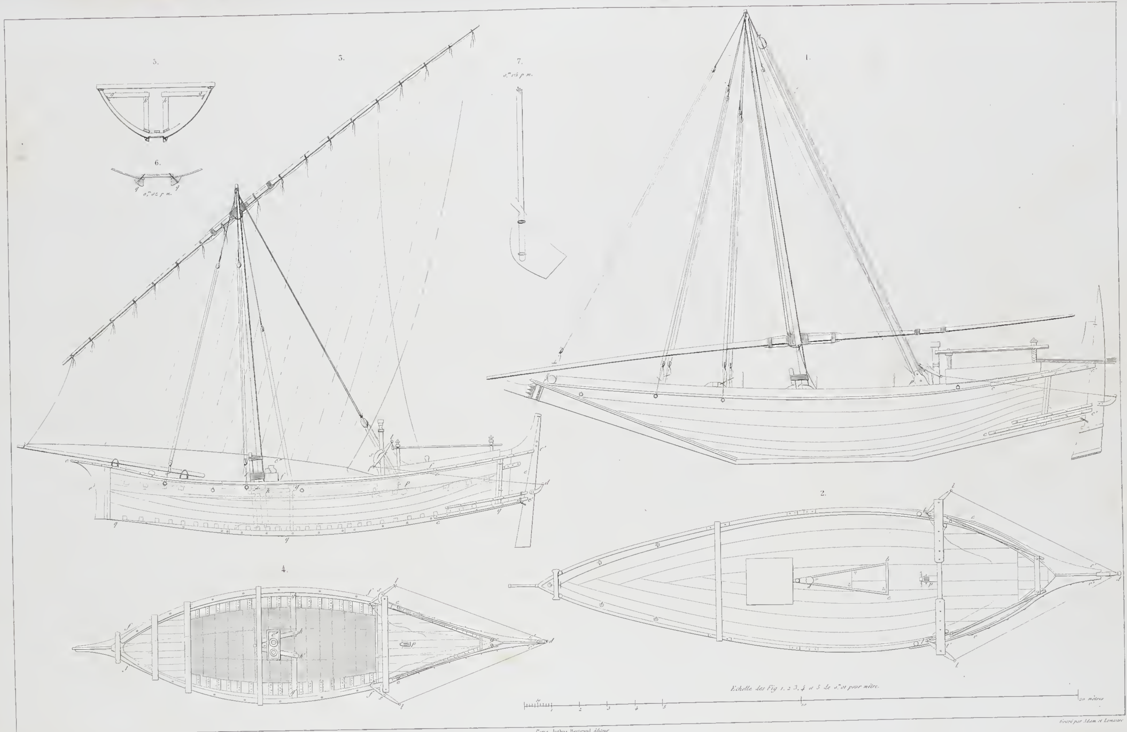
1. Ghazal de Mascate 2. Plan 3. Bedouin, grand bateau de pêche de Mascate 4. Plan 5. Section verticale par le maître bau 6. Détail de jonction des quilles et des bordages 7. Ancre.
