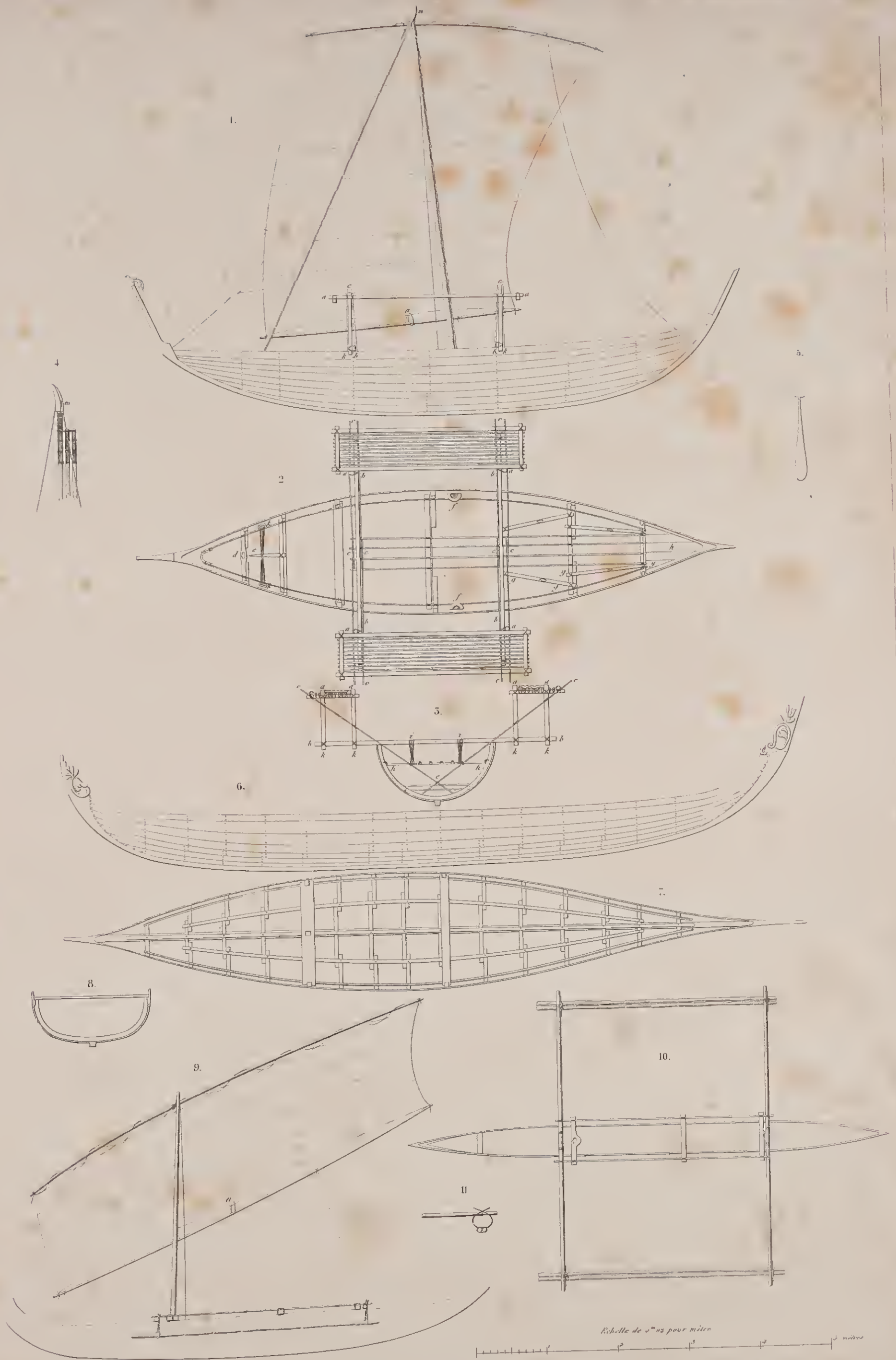
1. Bateau de pêche d'Amboine. 2. Plan. 3. Section. 4. Assemblage des trois mâts. 5. Péque. 6. Bateau employé à la pêche à la Seine. 7. Plan. 8. Section. 9. Péque d'Amboine. 10. Plan. 11. Section des balanciers aux leviers.
