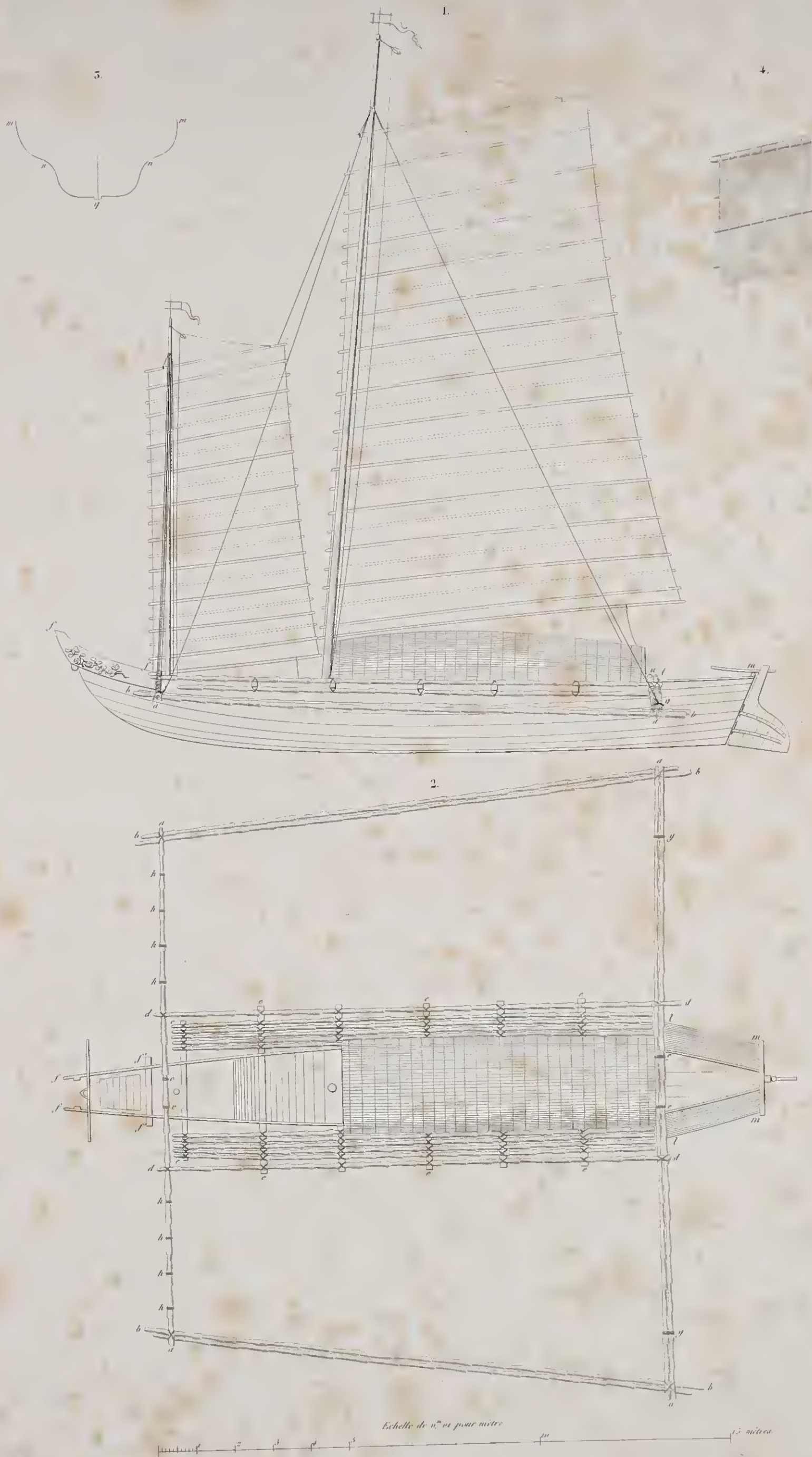
1. Catolador de la Laguna. 2. Plan. 3. Sección approach d'un Bidatto de la rivière de Stupit 4. Plan des vestes
