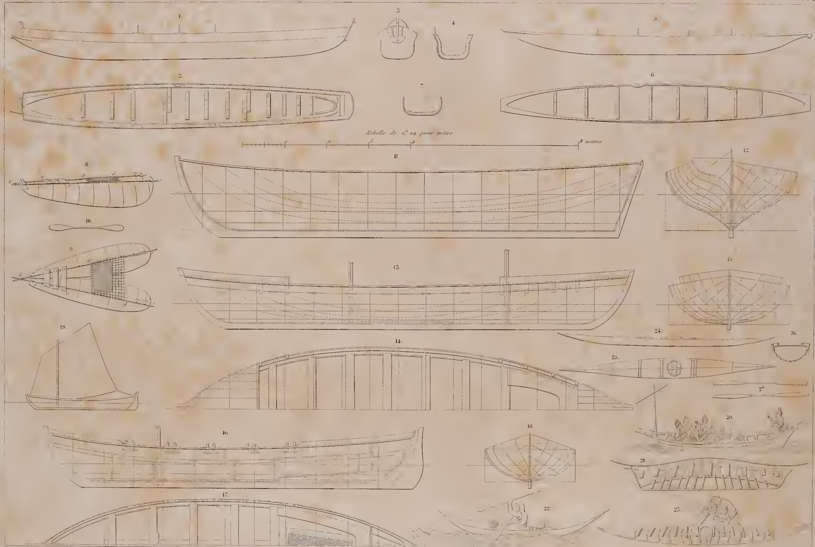
Plans des 1. Pirogue de Ulluar de l'Alme 2. Plan 3. Elevation de l'arrière. 4. Section. 5. Autre Pirogue de Ulluar 6. Plan 7. Section 8. Batse des paterneches 9. Plan 10. Pique. 11. Pirogue de Monté Ullur nommée l'Alme 12. Section. 13, 14, 15, 16, 17, 18 et 19. Batse de Monté Ullur 20. Homme en bateau de femme du Groenland. 21. Caroupe. 22. Homme en bateau de pêche du Groenland. 23. Caroupe 24. Homme (musée) au musée naval. 25. Plan 26. Section 27. Pique. Les fig. 12, 13, 14, 15, 16, 17, 18 et 19 sont esquissés d'après des plans de M. Roger, ingénieur de la marine.
