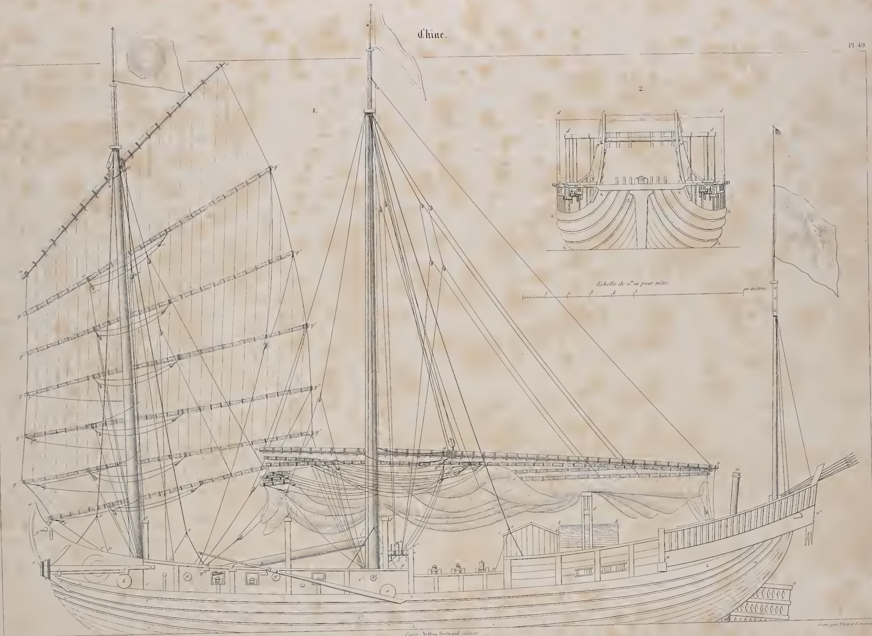
1. Grande Jonque de guerre. 2. Elevation de l'avant
