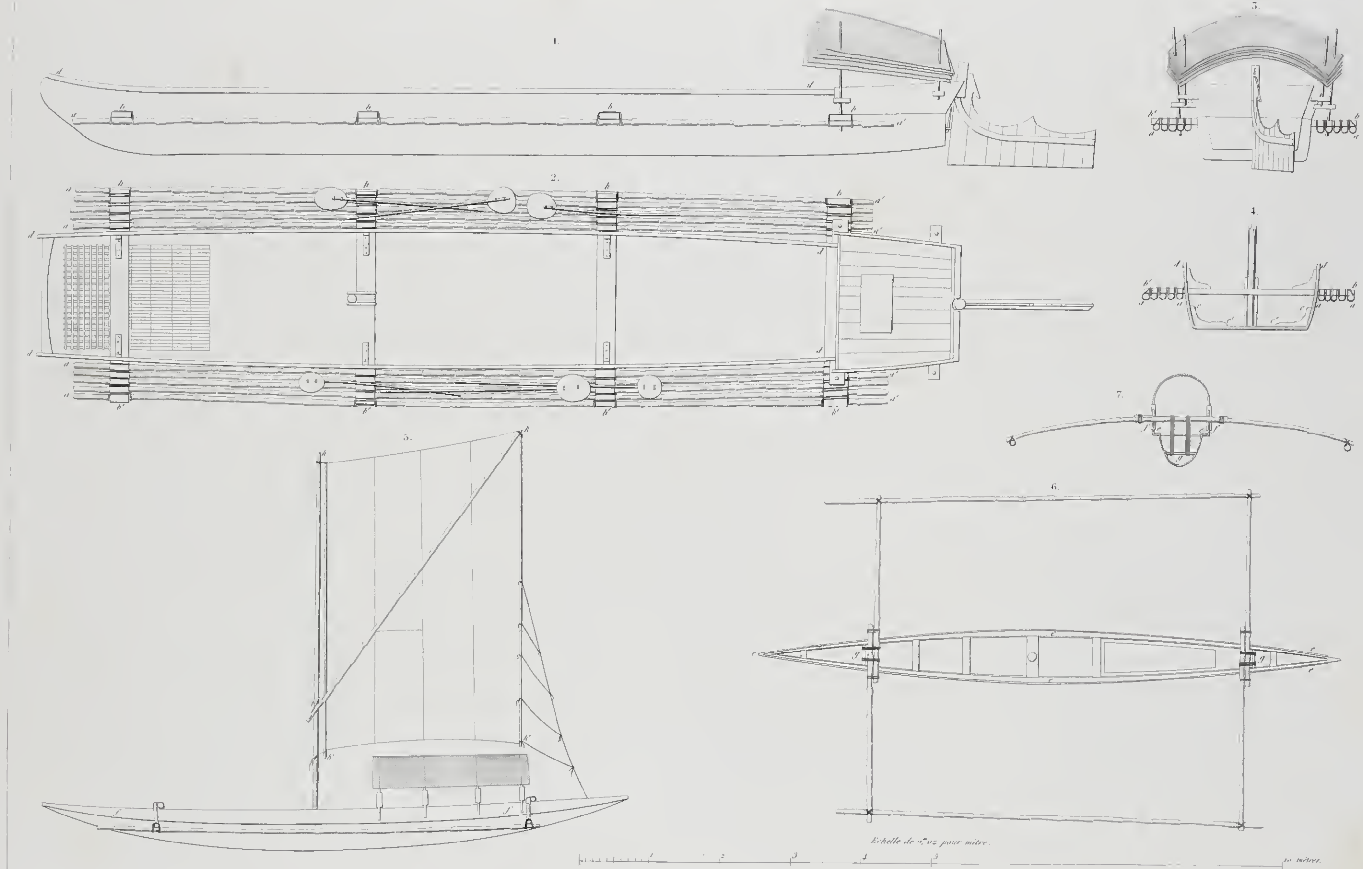
1. Casse, bateau de transport de Manille. 2. Plan. 3. Elevation de l'arrière. 4. Section. 5. Pirogue à double balancier de la Laguna. 6. Plan. 7. Section.
