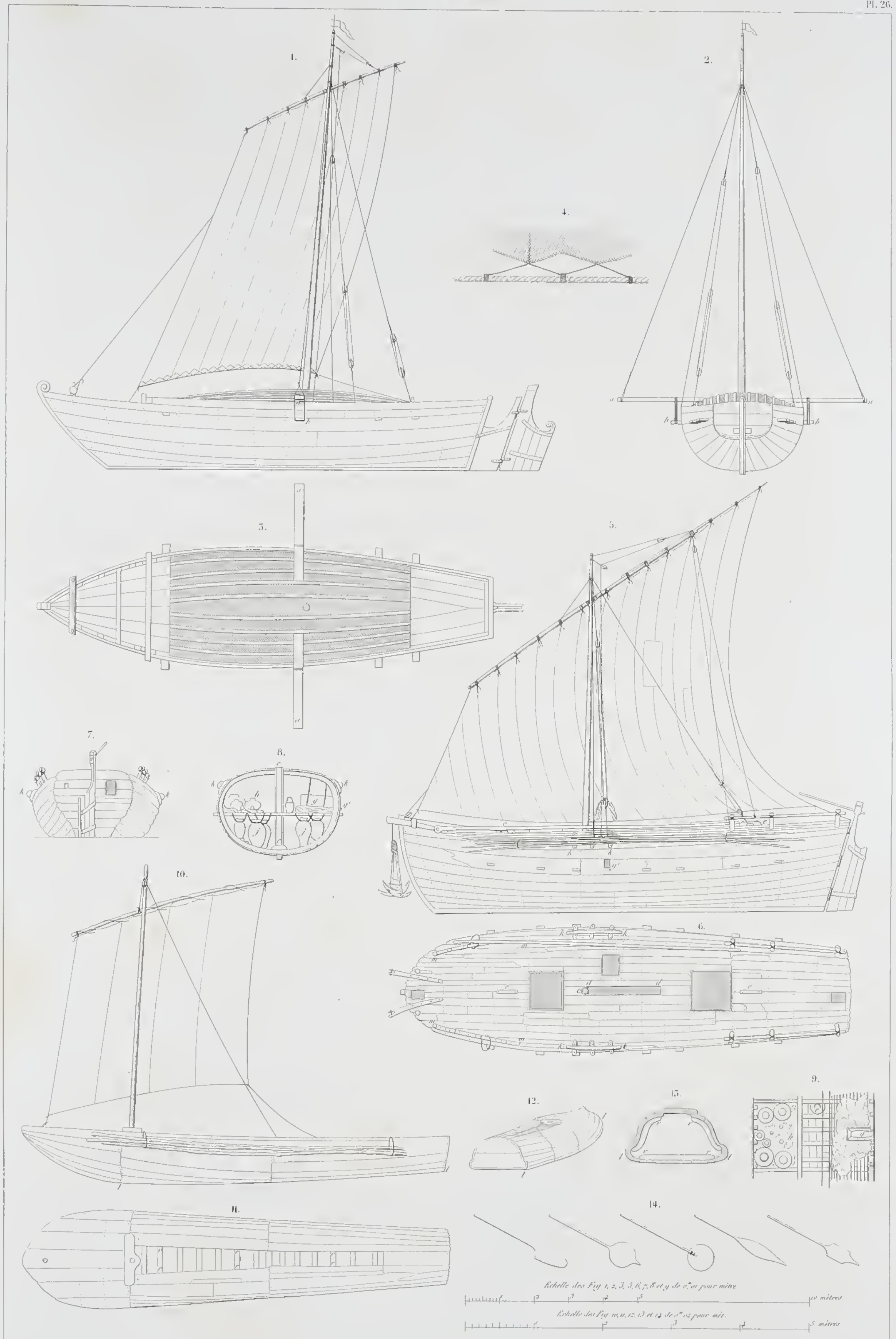
1. Petit caboteur de la côte de Coromandel. 2. Elevation par l'arrière. 3. Plan. 4. Manière dont la voile est ratinée. 5. Caboteur de la pointe de Devi. 6. Plan. 7. Elevation de l'arrière. 8. Section par le grand mât. 9. Plan de la platte-forme int. qui sert de cuisine. 10. Bateau souchier de Coromandel. 11. Plan. 12. Vue par l'arrière. 13. Vue par le mât. 14. Diverses pagaies.
