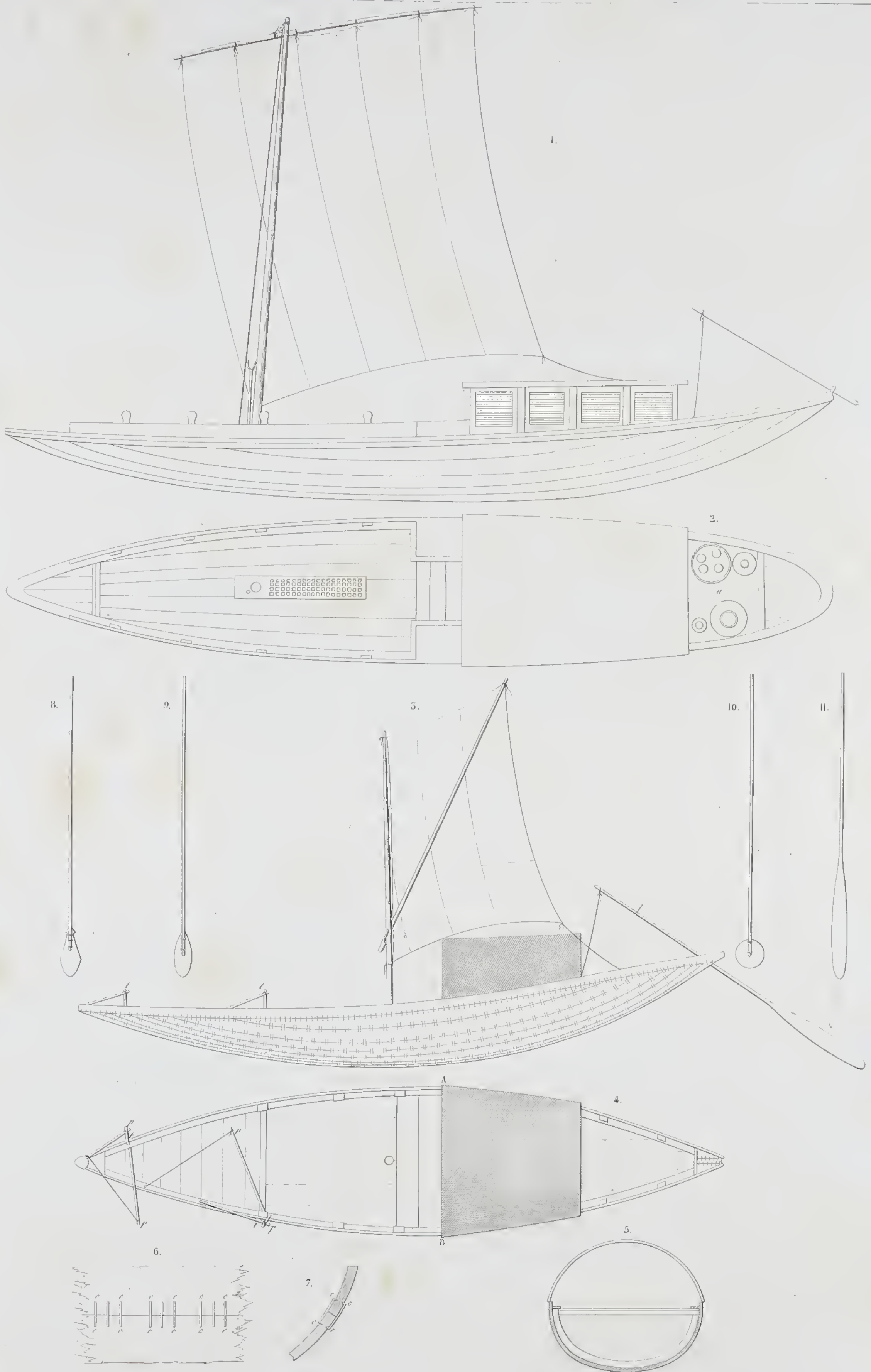
1. Petit Baulak. 2. Plan. 3. Dinghy. 4. Plan. 5. Section par A B. 6. Manière dont sont unis les bordages sous de pices. 7. id de pice. 8, 9, 10 et 11 Divers. Armes usées dans le pays.
