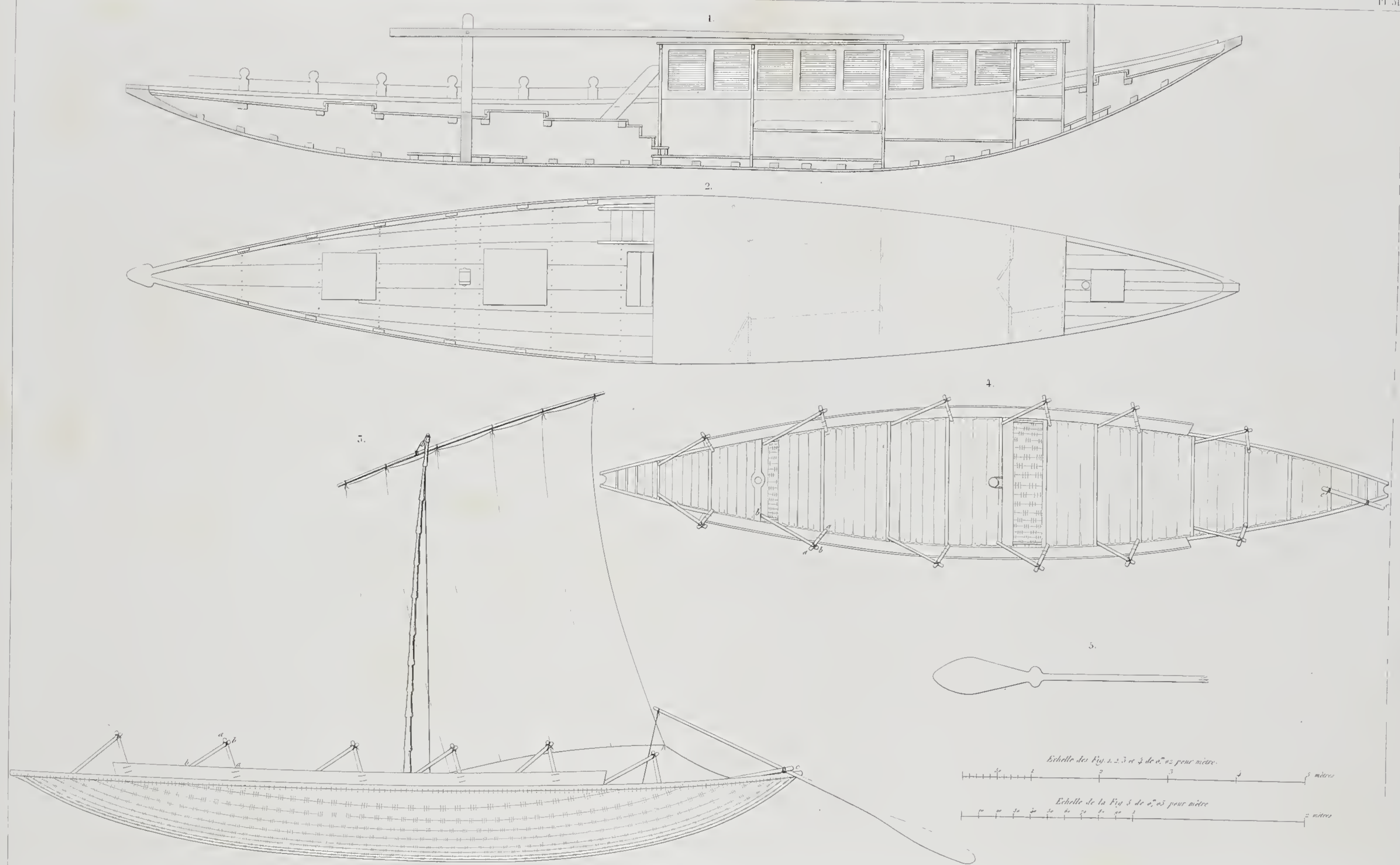
1. Section longitudinale d'un grand Boutein en l'état de passage 2. Plan. 3. Boutein indien des bouches du Gange. 4. Plan. 5. Aviron.
