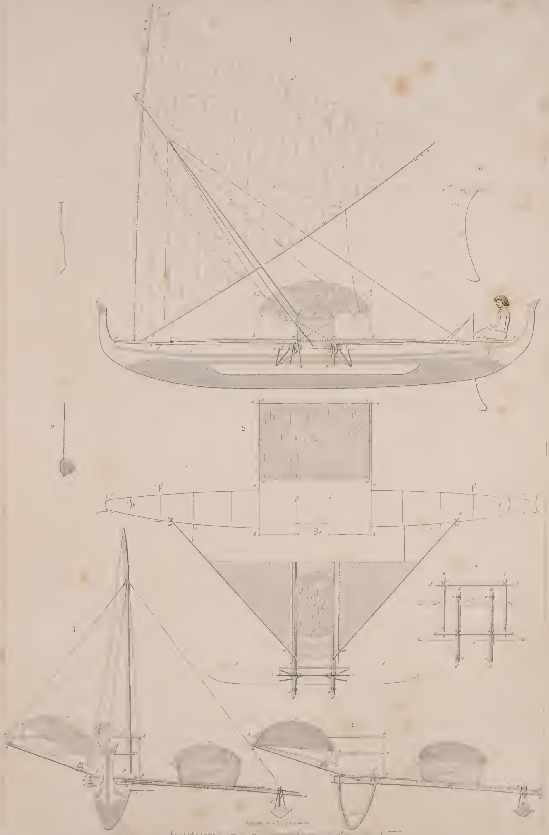
1 Vue de l'extérieur 2 Plan 3 Elevation de l'intérieur 4 Section par le milieu 5 Plan de la charpente qui soutient les deux côtés 6 Gouvernail 7 Rames 8 Coup
