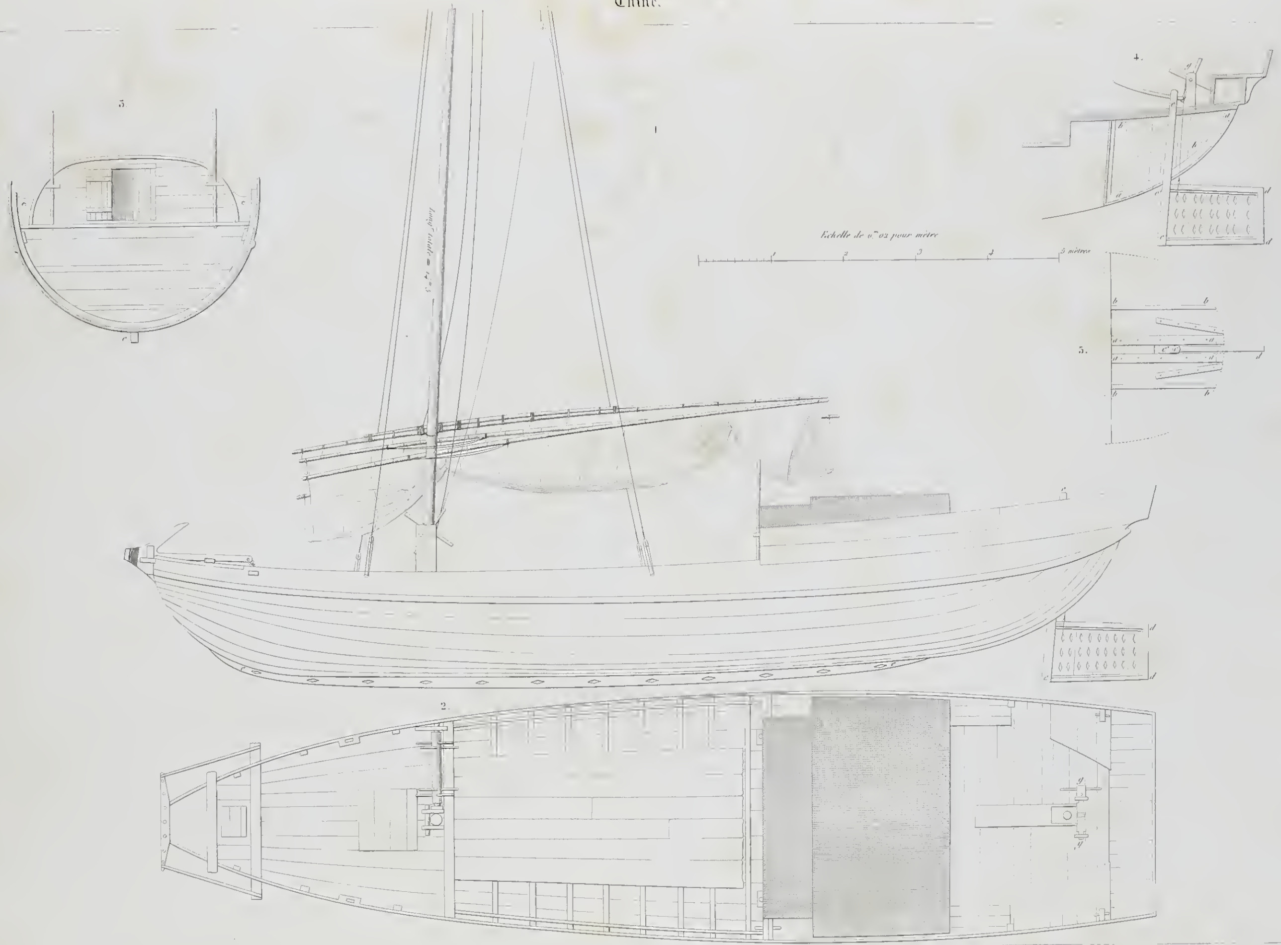
Figure 1. Petit bateau de transport de l'Huac. 2. Plan 3. Section par le maître bau 4. Section longitudinale de l'arrière 5. Plan de la chambre du gouvernail
