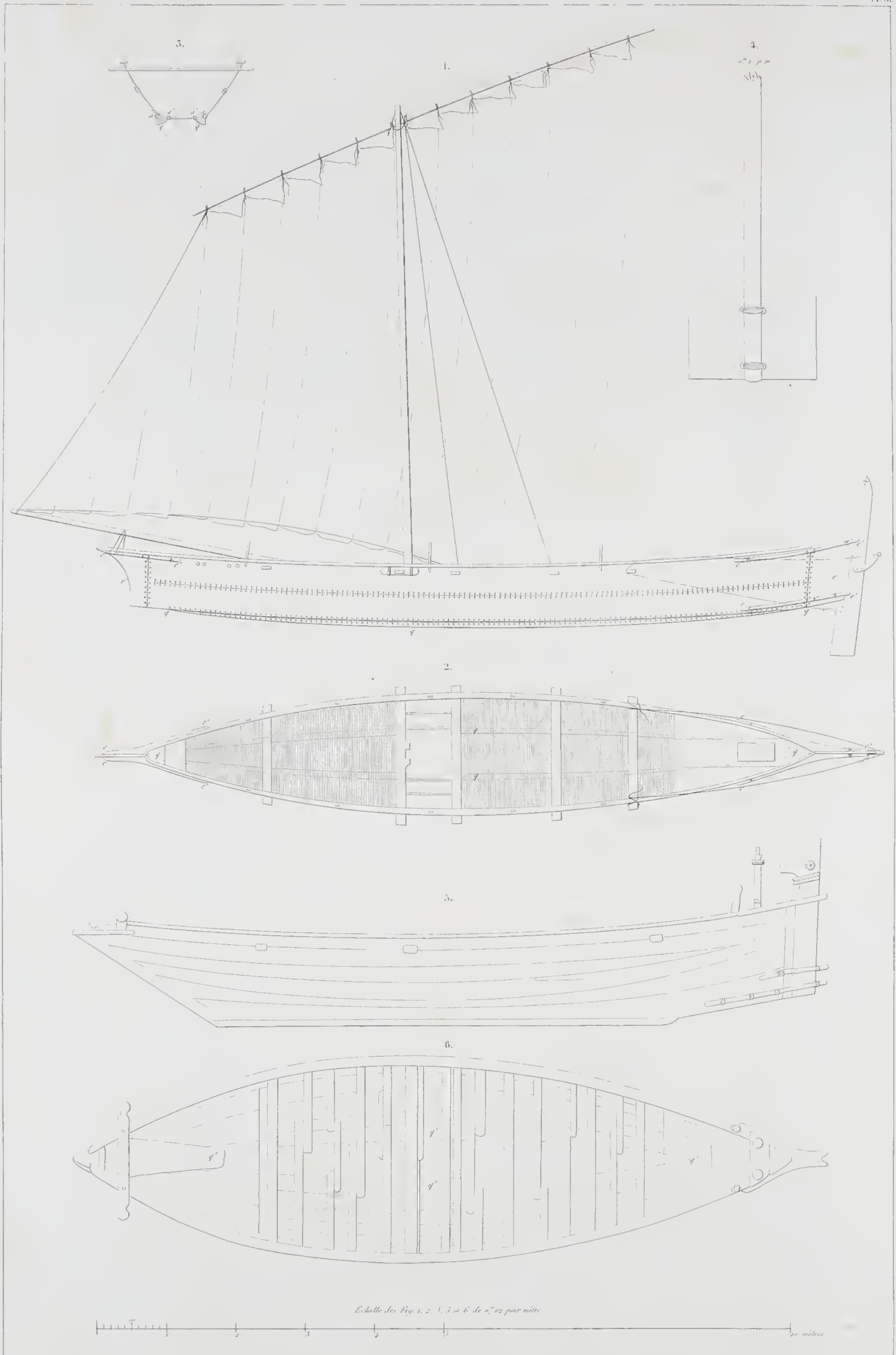
1. Petit bateau de pêche de Mascate nommé Biden-segal 2. Plan. 3. Section suivant le maître bau. 4. Stern 5. Bateau de charge de Mascate nommé Biden-mutt-kumal 6. Plan.
