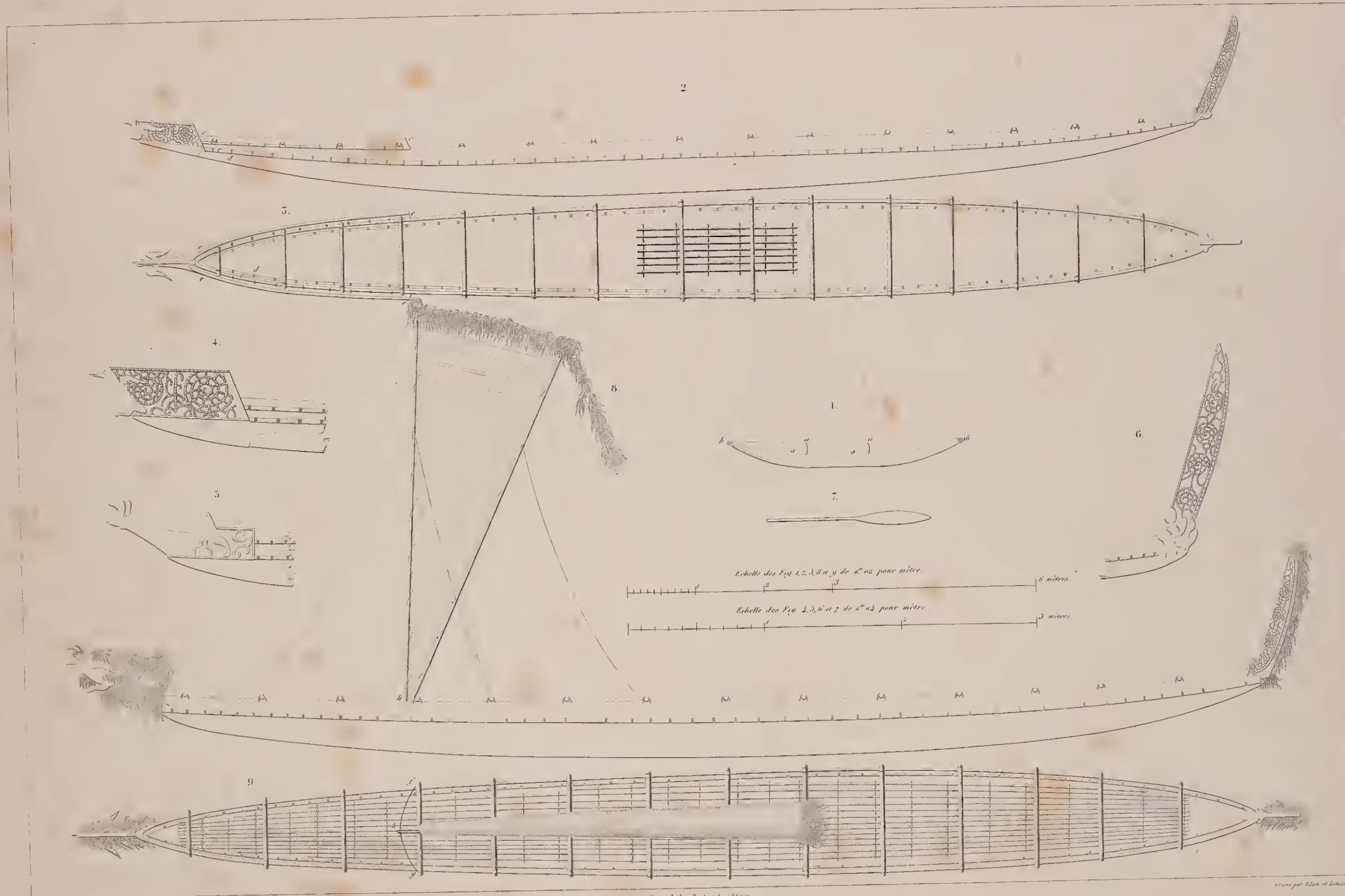
Paris del. Paris Art. Berthoud, éditeur. 1. Canoe en corce de la baie Jervis. 2. Canoe de l'anse de l'Islet de l'île de Tuvai. 3. Canoe de l'anse de l'île de Tuvai. 4. Canoe de l'anse de l'île de Tuvai. 5. Canoe de l'anse de l'île de Tuvai. 6. Canoe de l'anse de l'île de Tuvai. 7. Canoe de l'anse de l'île de Tuvai. 8. Canoe de l'anse de l'île de Tuvai. 9. Canoe de l'anse de l'île de Tuvai.
