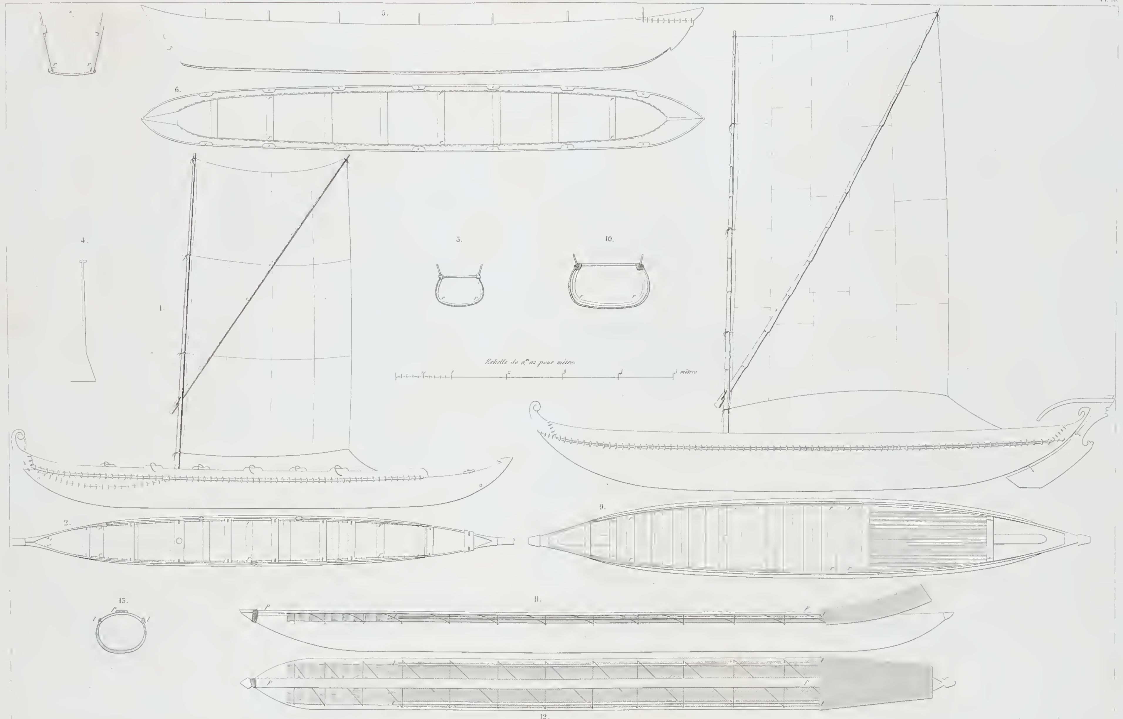
I. Proque de Malé 2. Plan 3. Section 4. Laque 5. Bateau plat de Calicut 6. Plan 7. Section 8. Bandar manché bateau de charge de Cichin 9. Plan 10. Section 11. Proque de la rivière de Calicut, employée au transport du riz 12. Plan 13. Section
