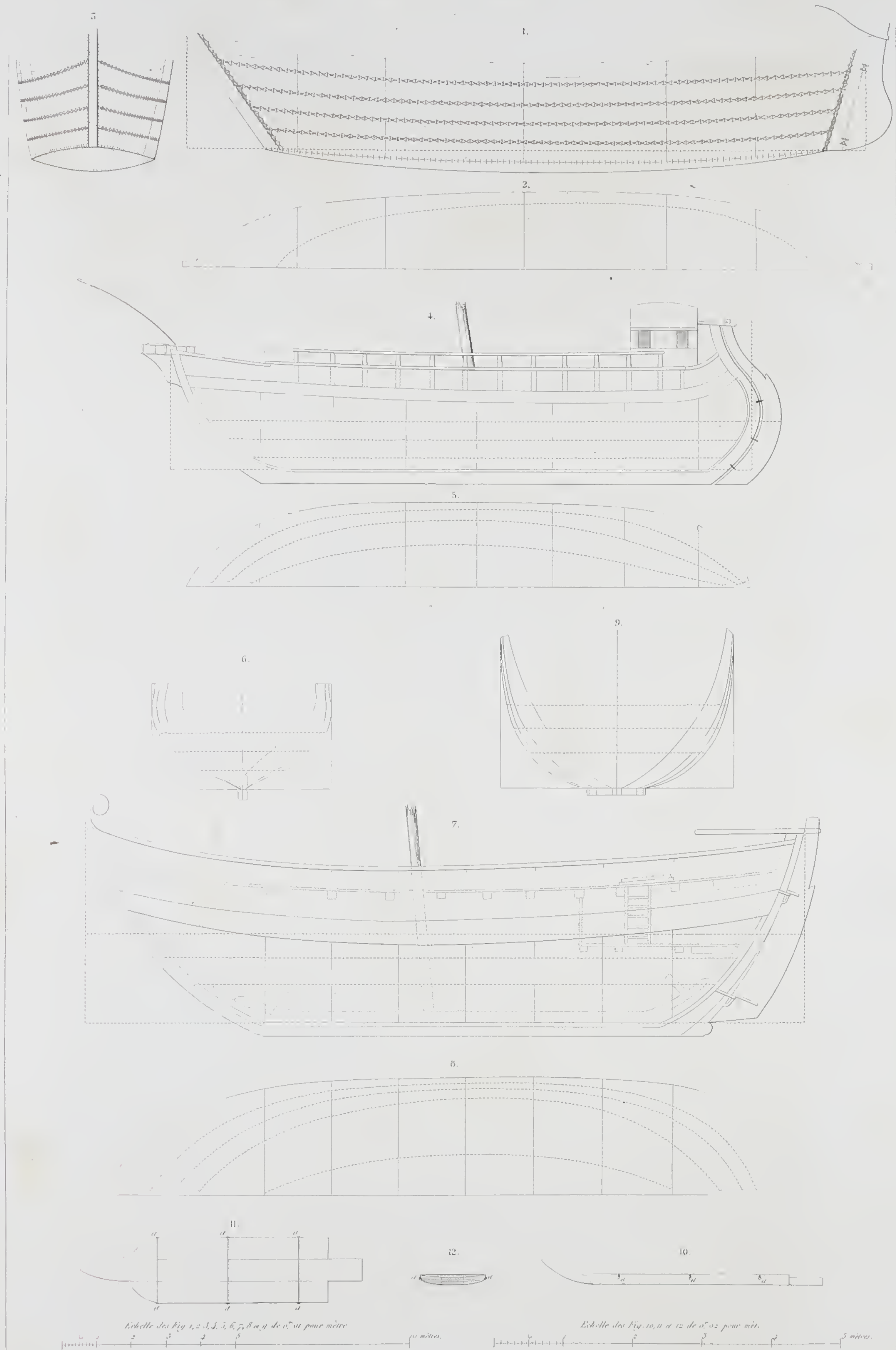
Plan de la 1. Manche de Mangrove 2. Plan 3. Croisement de l'arc 4. Profil 5. Plan 6. Section 7. Plan 8. Plan 9. Section 10. Colonne du golfe de Manar nommé 'Lepan' 11. Plan 12. Section
