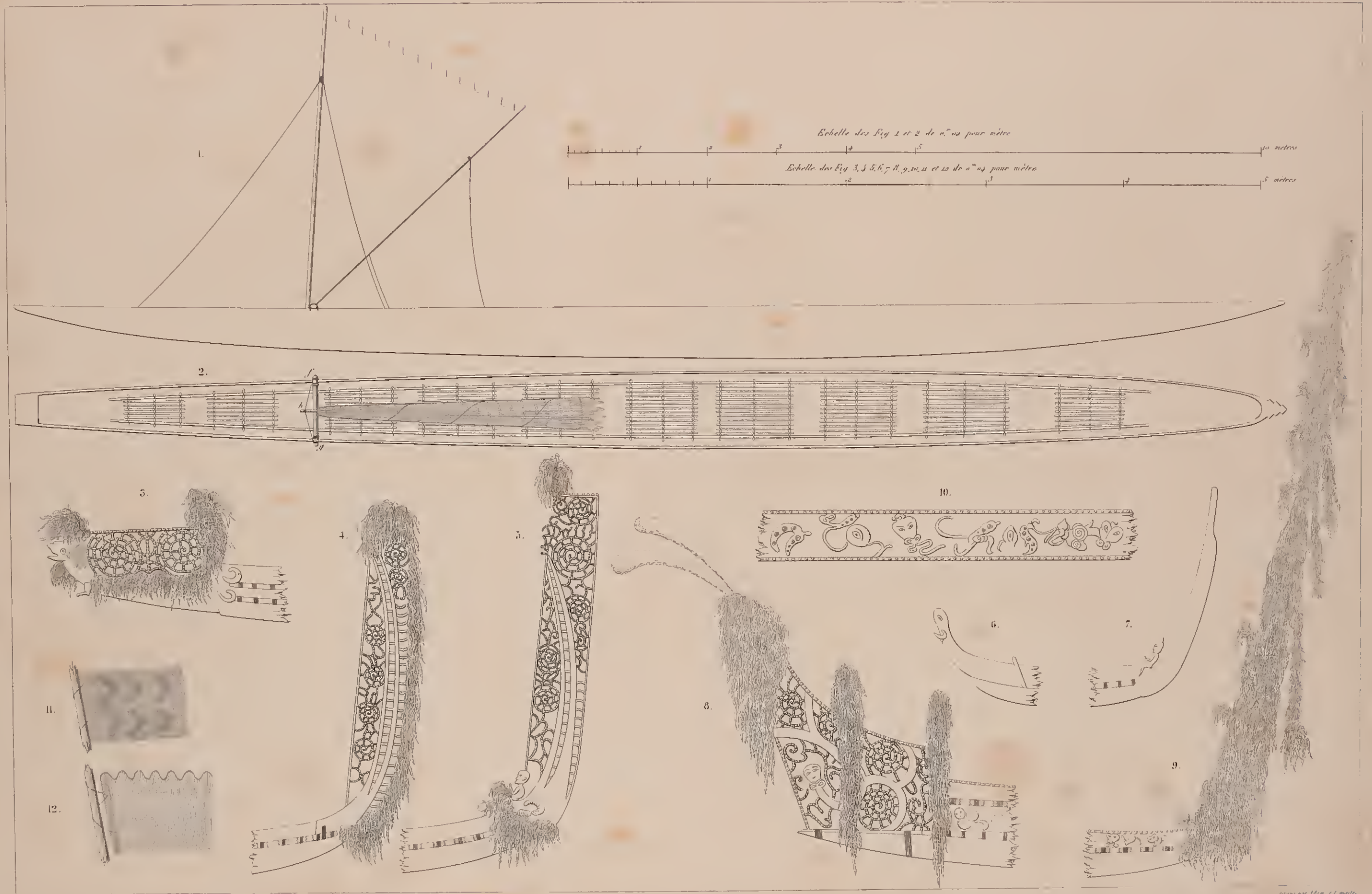
1. Voûte de la baie - Wharangi dans l'île - Whana - Hauri 2. Plan. 3, 4, 5, 6 et 7. Ornements de Voûtes de la baie - Whana-hana 8. Devant d'une grande Voûte de la baie - Whangara 9. Ornement de l'arrière 10. Sculpture de la poutre 11 et 12. Seprés de voûtes
