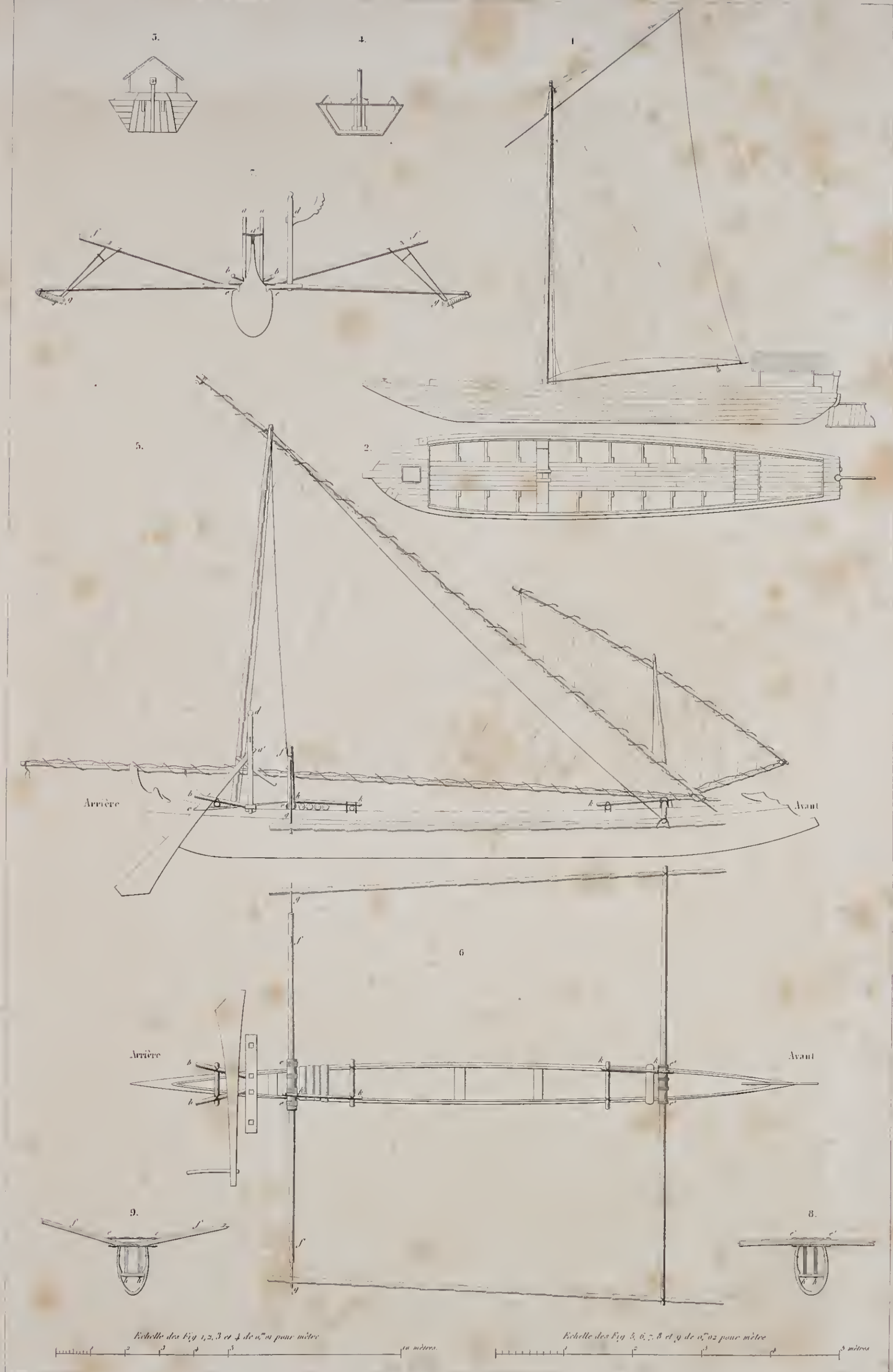
1. Grand bateau de transport de Batavia. 2. Plan. 3. Elevation de l'arrière. 4. Section. 5. Plan d'endurance de Batavia. 6. Plan. 7. Elevation de l'arrière. 8. Section par le tiers de l'avant. 9. idem par celui de l'arrière.
