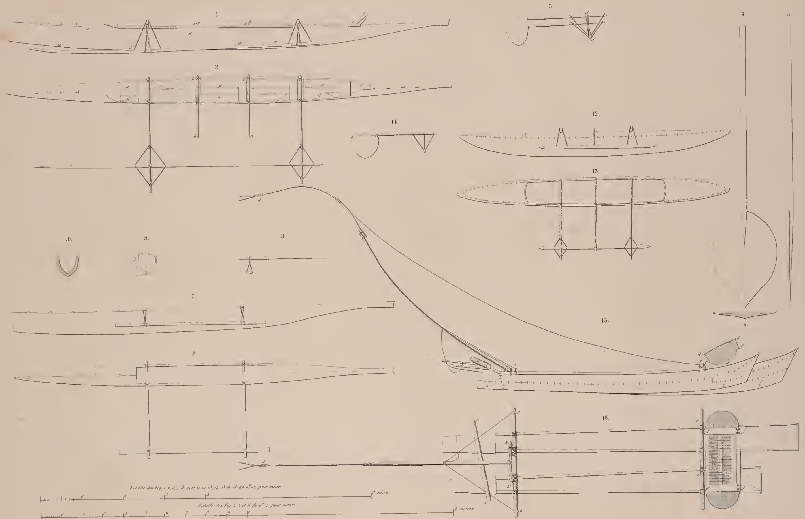
1. Tupahunga de Tonga - Tabou 2. Plan 3. Elevation de l'avant 4. Rigage de face 5. et de profil 6. Autre 7. Petite Tupahunga 8. Plan 9. Détails divers 10. Croquis 11. Déposition du balancier 12. Pirogue grossièrement construite nommée Bepua 13. Plan 14. Elevation de l'avant 15. Pirogue double de Taïti servant à la pêche au flambeau 16. Plan
