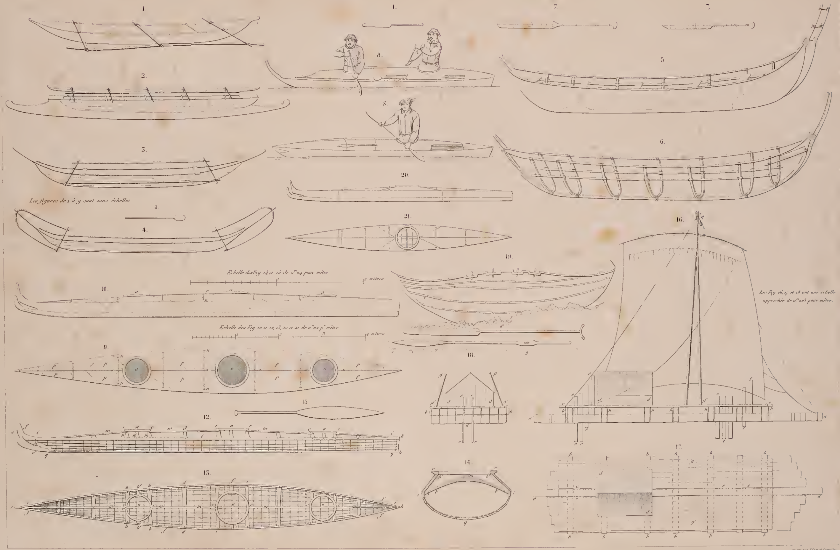
1 et 2. Pirogues de l'île Kamanzoff (Archipel Pé-Melou). 3 et 4. Bateaux à rames de l'île de Niquis. 5. Bateau en peau de l'île St-Laurent (Nes Alentiennes). 6. Charpente. 7. Pirogues. 8 et 9. Baydargues d'Oronishka. Côte N.O. d'Amérique. 10. Baydargue de Berdiga. 11. Plan. 12. Charpente intérieure. 13. Plan. 14. Section par le centre du grand trou d'homme. 15. Pirogue. 16. Balsa en fongula de Gungaguit. 17. Plan. 18. Vue de l'avant. 19. Canot du Nantichka. 20. Baydargue de Berdiga, à une place. 21. Plan. (Les figures 1, 2, 3, 4, 5, 6 et 7 sont tirées du voyage du Cap Kotzebue.)
